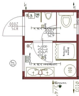
10' Sanitär-Container
