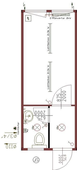
20' Büro mit WC-Abteil
