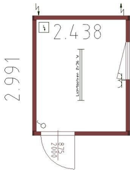
10' Büro
