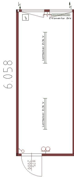
20' Büro
