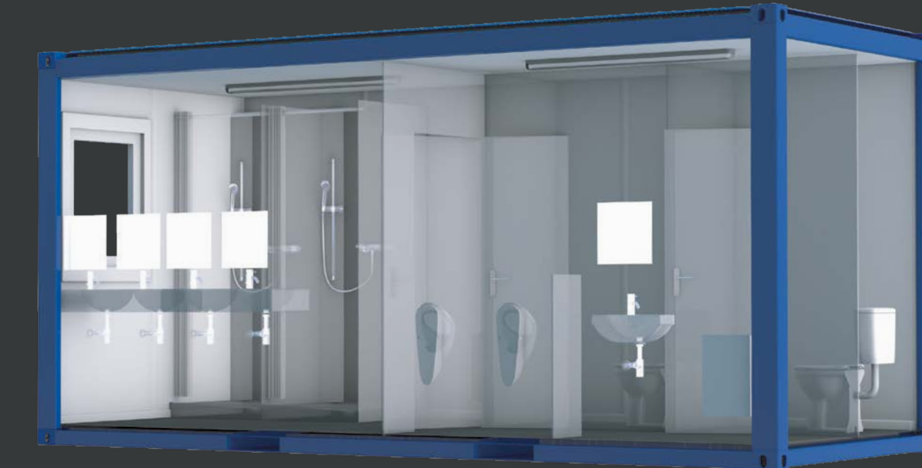
SA6 20' Damen/Herren WC-Container mit Pantry-Küche
