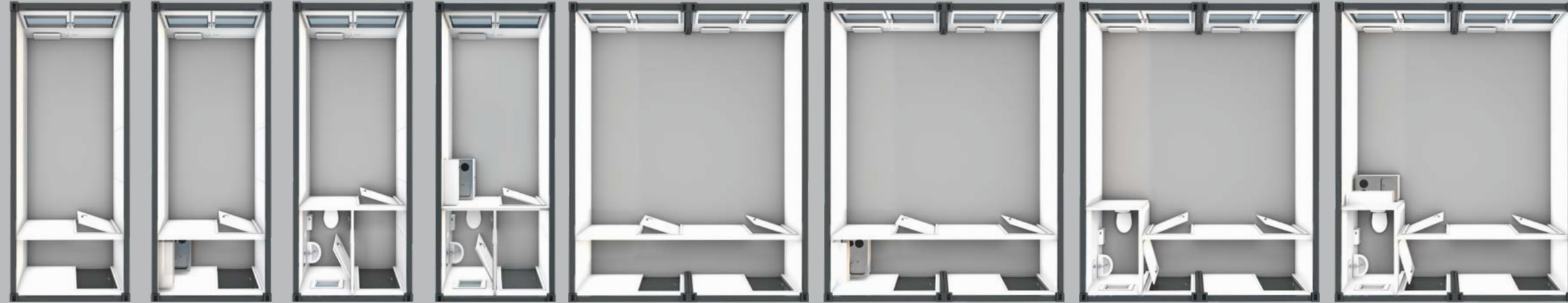
BM2 20' Raumcontainer BM3 20' Raumcontainer mit Pantry-Küche BM4 20' Raumcontainer mit WC-Abteil BM5 20' Raumcontainer mit Pantry-Küche und WC-Abteil BM6 20' Raumcontainer 2er-Anlage BM7 20' Raumcontainer 2er-Anlage mit Pantry-Küche BM8 20' Raumcontainer 2er-Anlage mit WC-Abteil BM9 20' Raumcontainer 2er-Anlage mit Pantry-Küche und WC-Abteil
