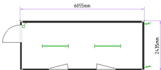
Bürocontainer 20'
