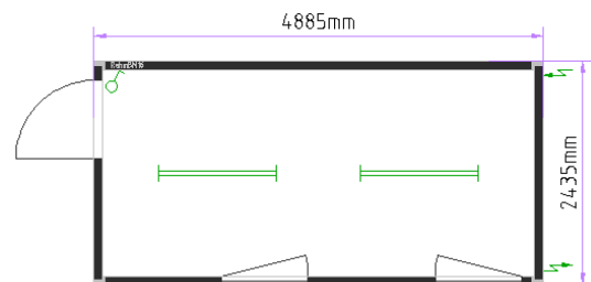
Bürocontainer 16'
