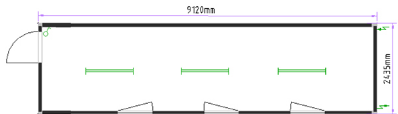
Bürocontainer 30'
