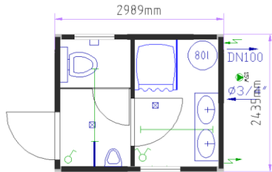
Sanitärcontainer 10'
